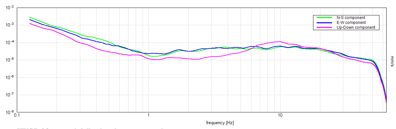
HVSR 38: spettri delle singole componenti
