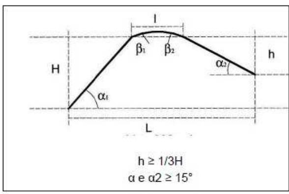
Fig. 9 - Criteri di riconoscimento delle creste e/o cocuzzoli suscettibili di amplificazioni morfologiche (v. all. A dgrv 1572/2013)
