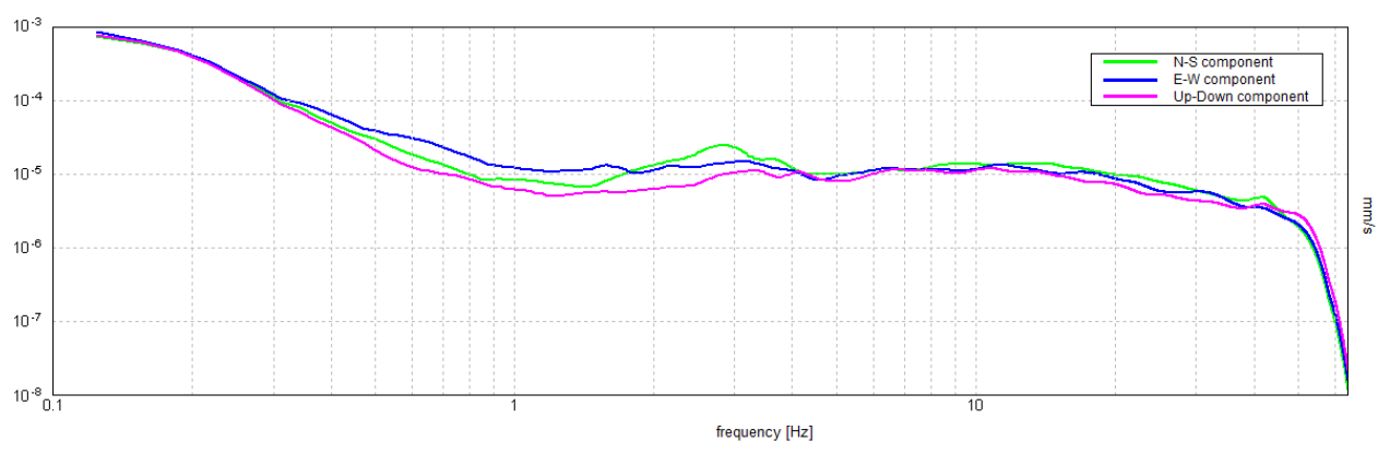
HVSR 36: spettri delle singole componenti
