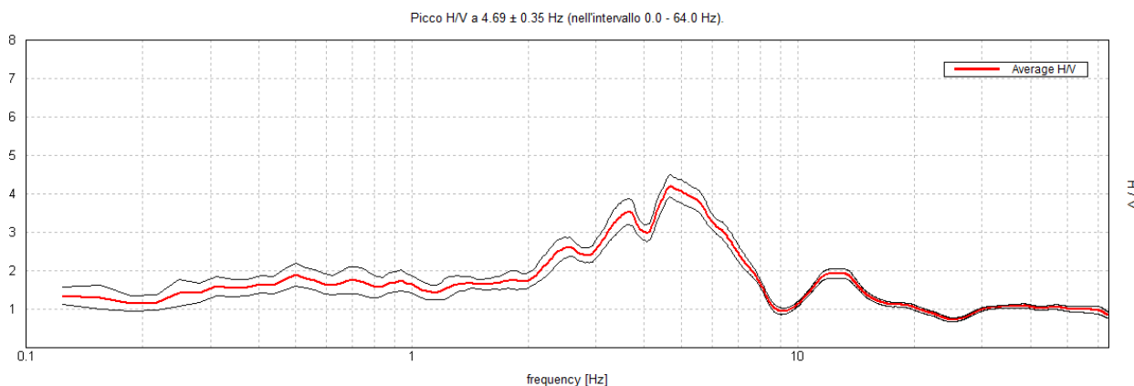
HVSR 35: rapporto spettrale H/V
