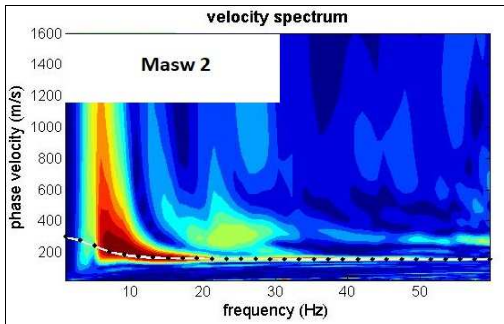
Spettro MASW 2
