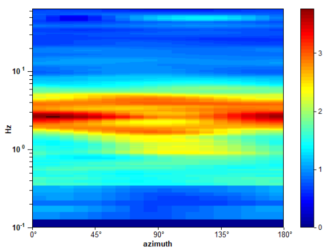
HVSr 37: direzionalità
