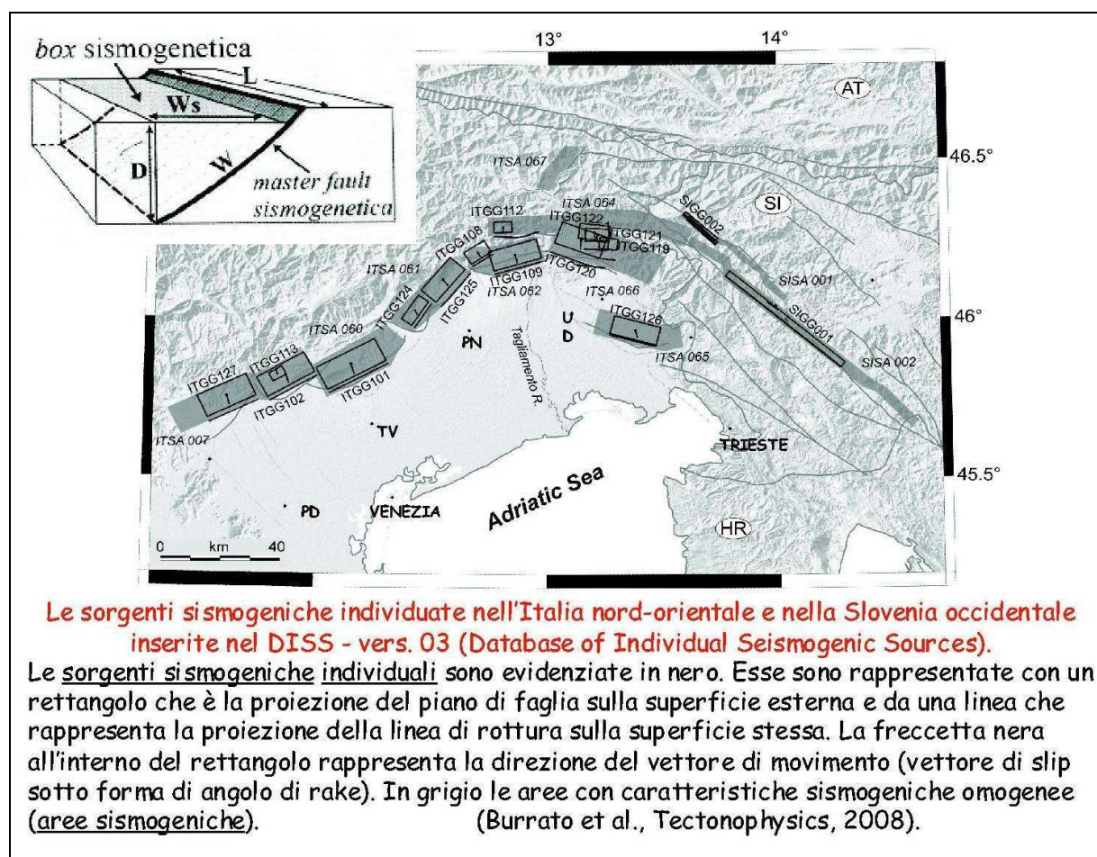
Fig. 4 - Sorgenti sismogenetiche dell'Italia Nord-Orientale (Buratto e altri 2008)
