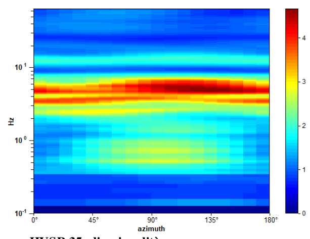
HVSR 35: direzionalità
