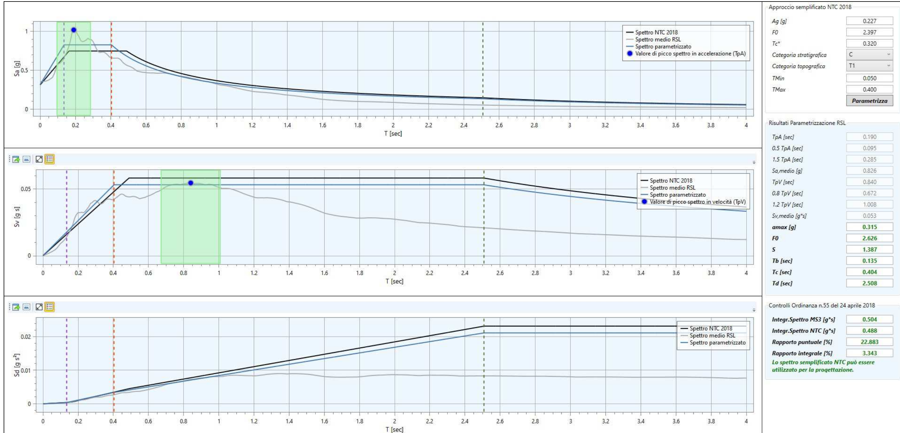
Fig. 13 – Confronto spettri di risposta medio RSL, NTC 2018, parametrizzato e valore di picco spettro in accelerazione nel punto di controllo P12 del sito in oggetto, in corrispondenza HVSr 36.
