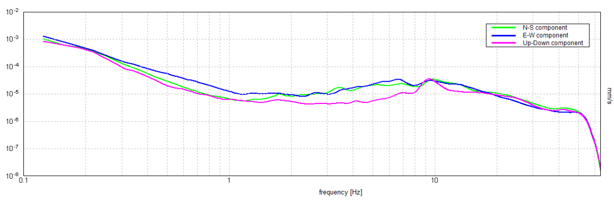
HVSR 35: spettri delle singole componenti
