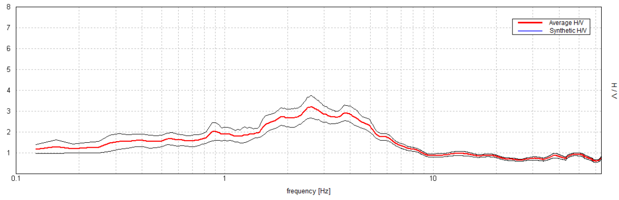
HVSR 37: rapporto spettrale H/V
