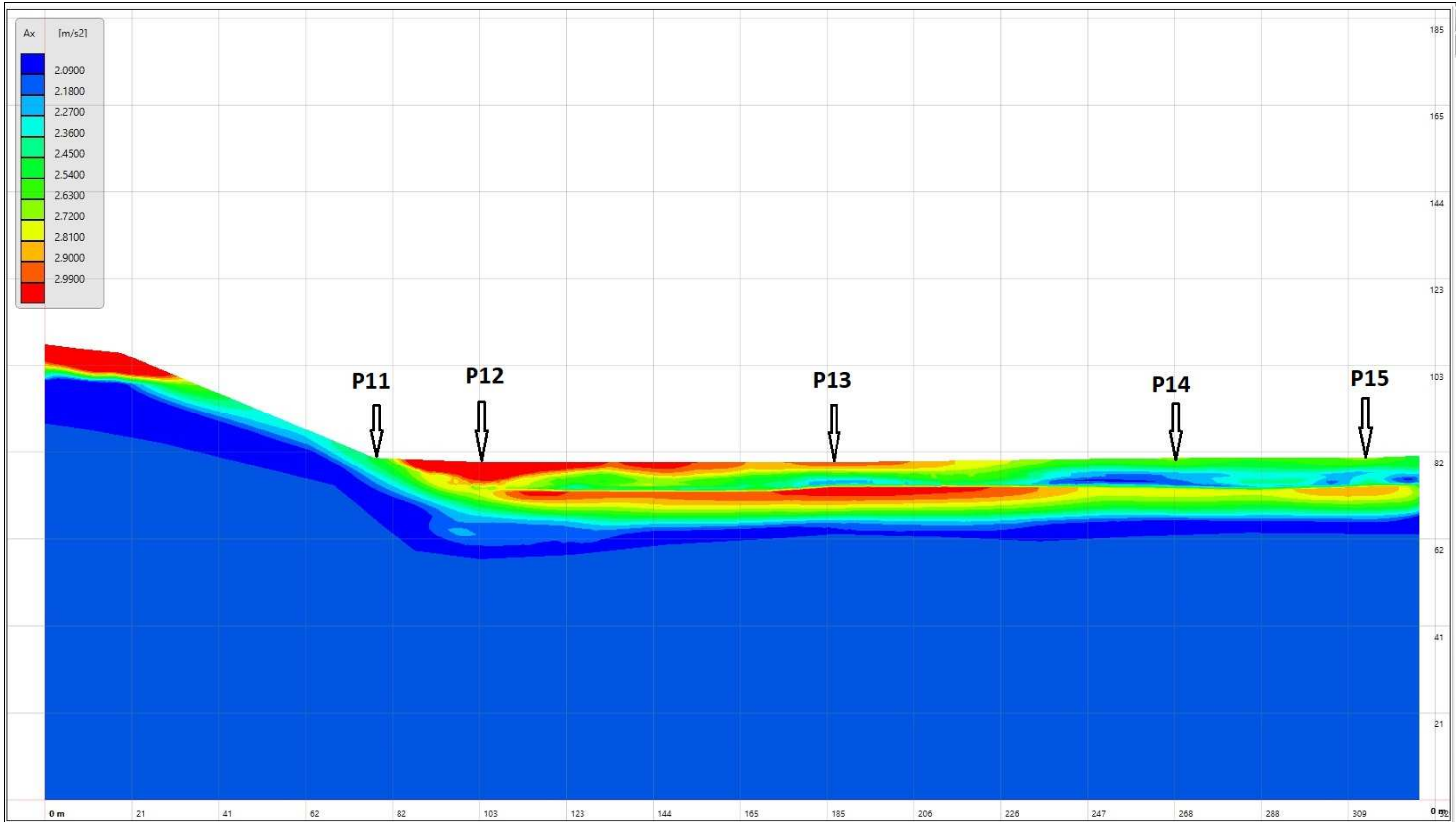
Fig. 11 -Calcolo di Risposta Sismica Locale: modello delle accelerazioni orizzontali lungo la sezione "A-B" (v. Tav.1)
