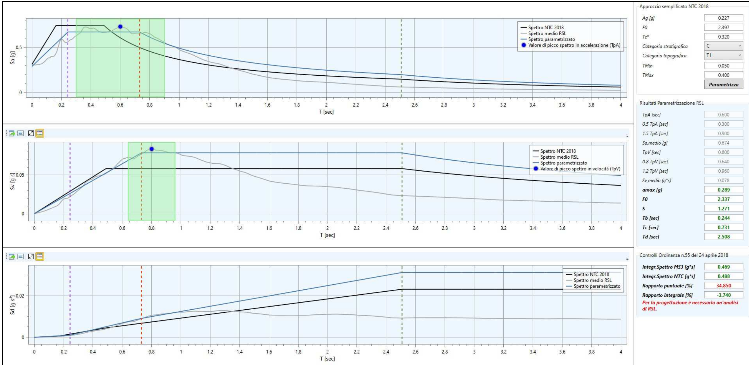
Fig. 14 – Confronto spettri di risposta medio RSL, NTC 2018, parametrizzato e valore di picco spettro in accelerazione nel punto di controllo P13 del sito in oggetto, in corrispondenza HVSR 37
