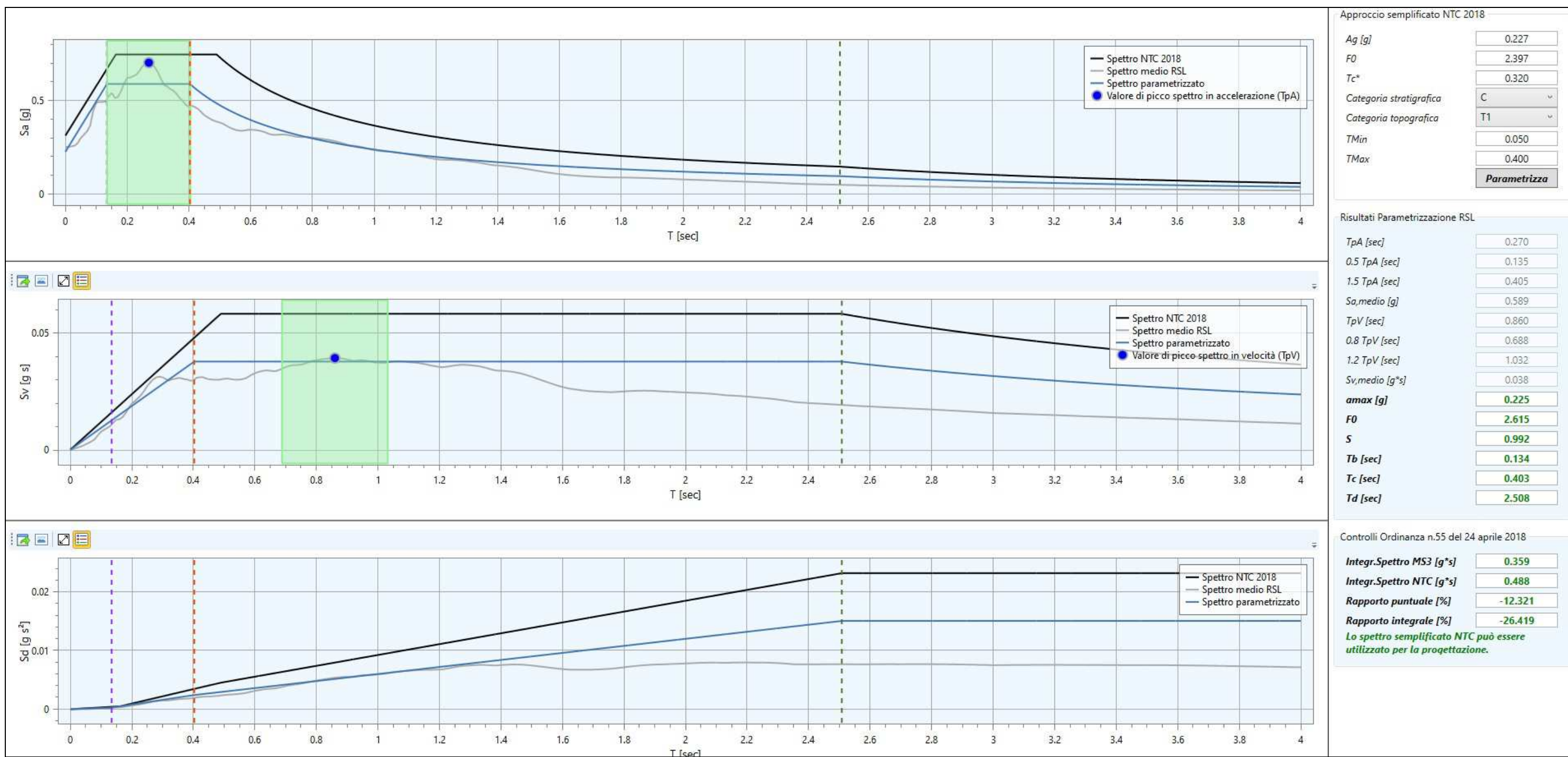
Fig. 12 – Confronto spettri di risposta medio RSL, NTC 2018, parametrizzato e valore di picco spettro in accelerazione nel punto di controllo P11 del sito in oggetto
