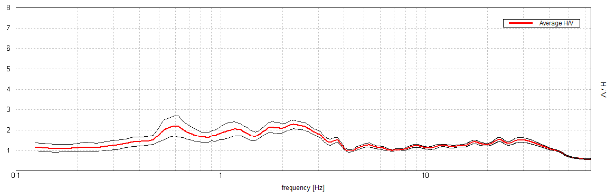
HVSR 36: rapporto spettrale H/V
