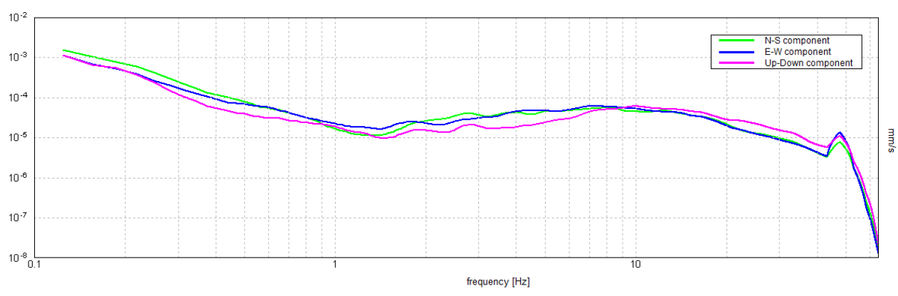
HVSr 37: spettri delle singole componenti
