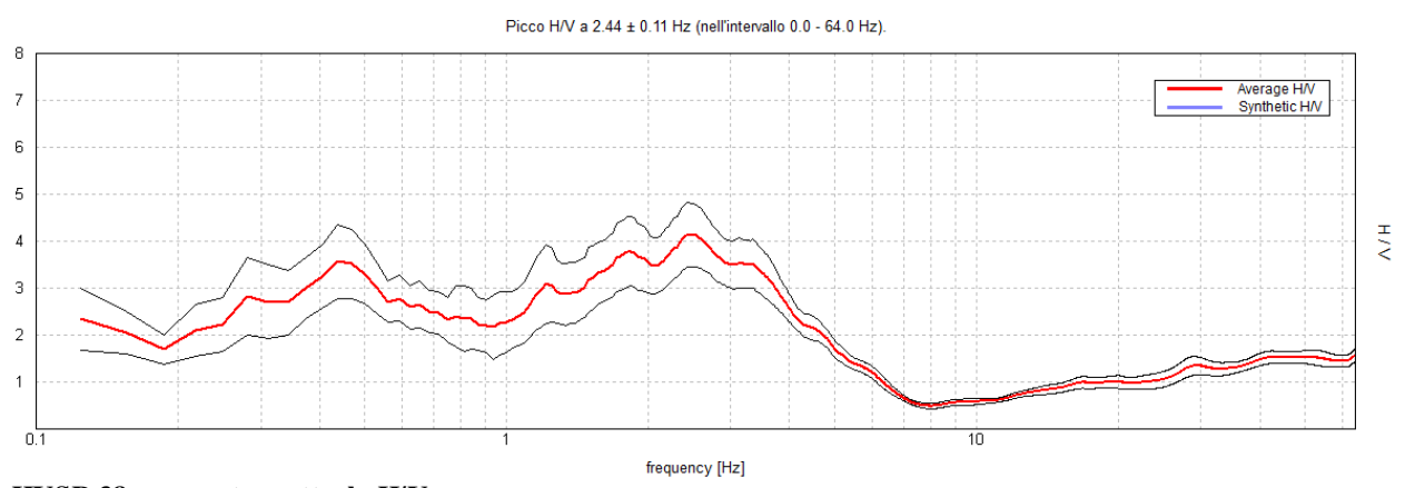
HVSr 38: rapporto spettrale H/V
