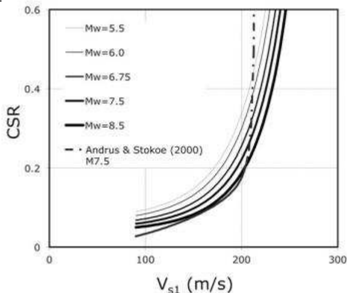
Fig. 17 – Grafico che evidenzia l'andamento delle curve, per valori di Mw da 5.5 a 8.5, in funzione di Vs1 e CSR (da Kayen e altri, 2013).
