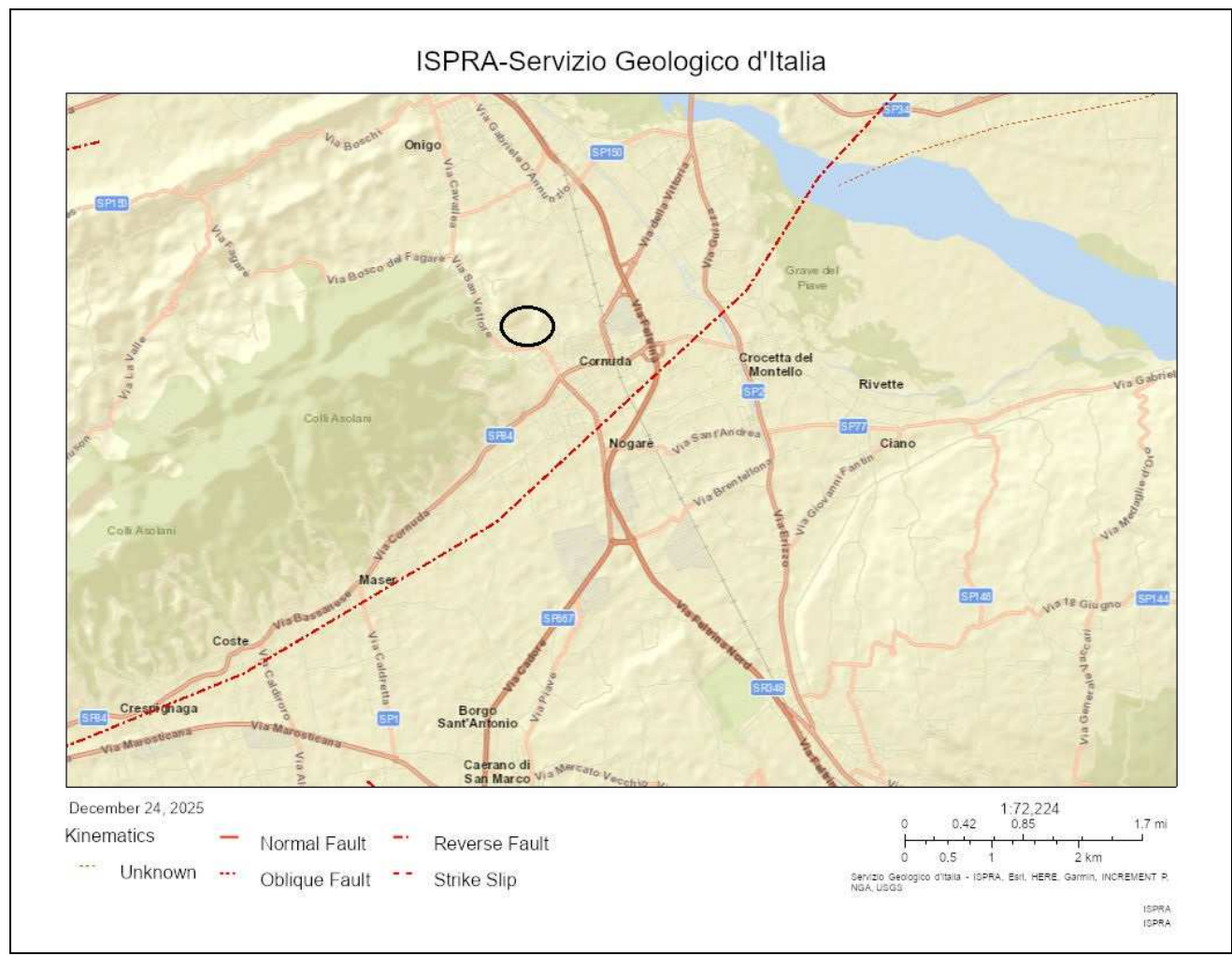
Fig. 6 - Faglie attive nell'area di Cornuda o limitrofa (progetto Ithaca - Italy Hazard from Capable Faults) – le linee verdi sono i confini comunali, quelle rosse/arancioni sono le faglie.
