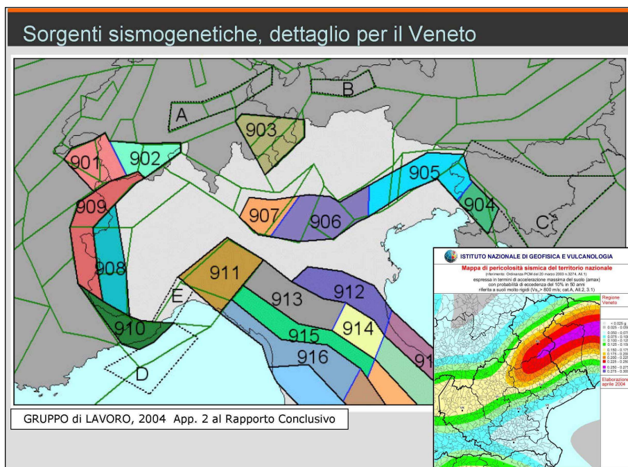
Fig. 5 - Zonazione sismogenetica ZS9 del Veneto
