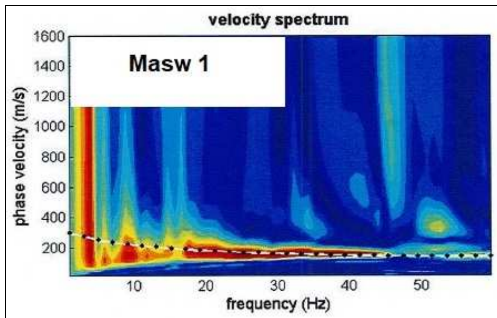
Spettro MASW 1
