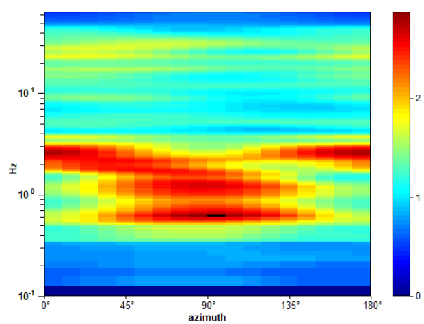
HVSR 36: direzionalità
